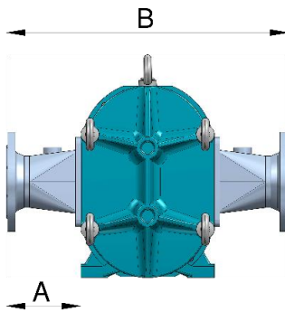
Baureihe 1 Anschlussstutzen mit Anschlussflansch und O-Ring in mm / inches Design 1 Short, straight pipe connectors with connection flange and O-ring seal in mm / inches
